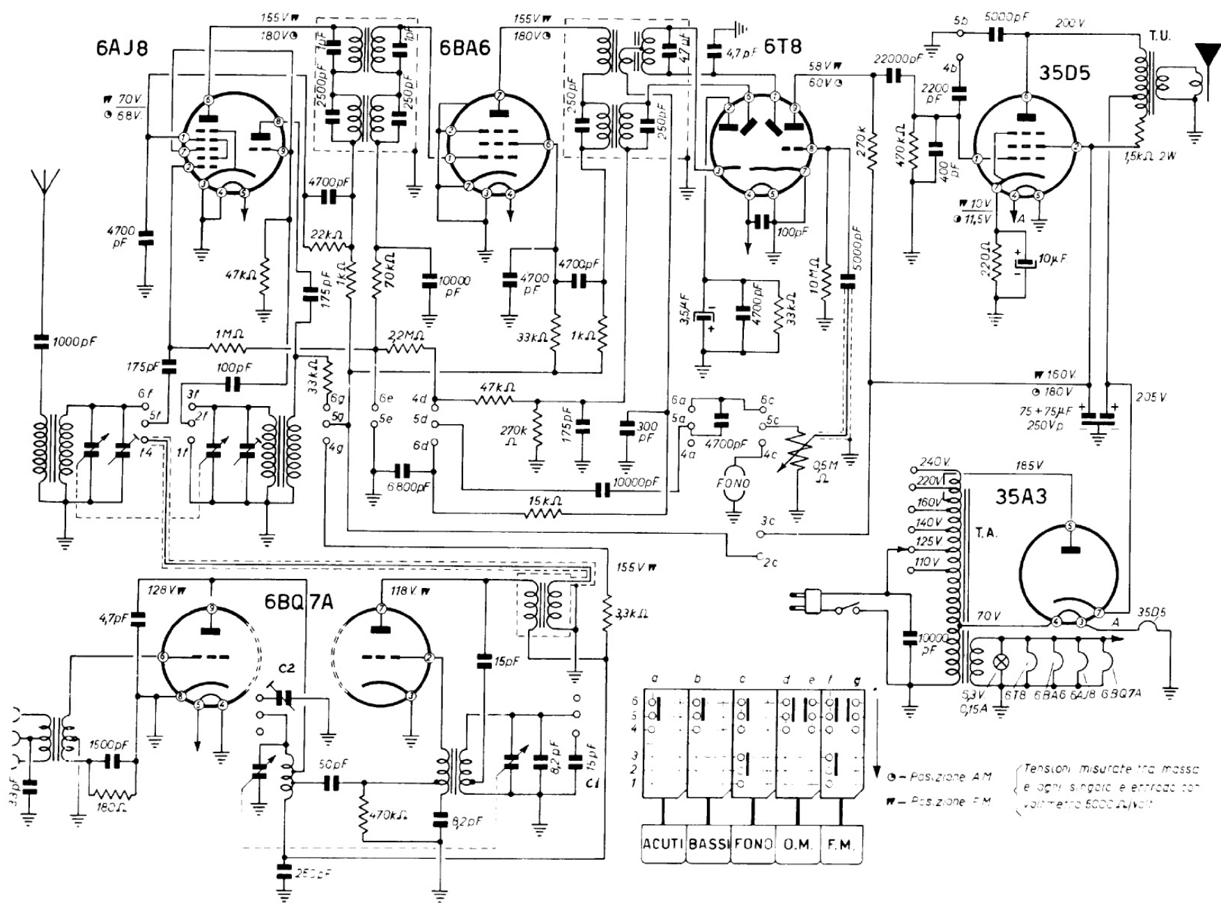
SCHEMA ELETTRICO DEL RADIORICEVITORE G.B.C. FM/200 GLADE
